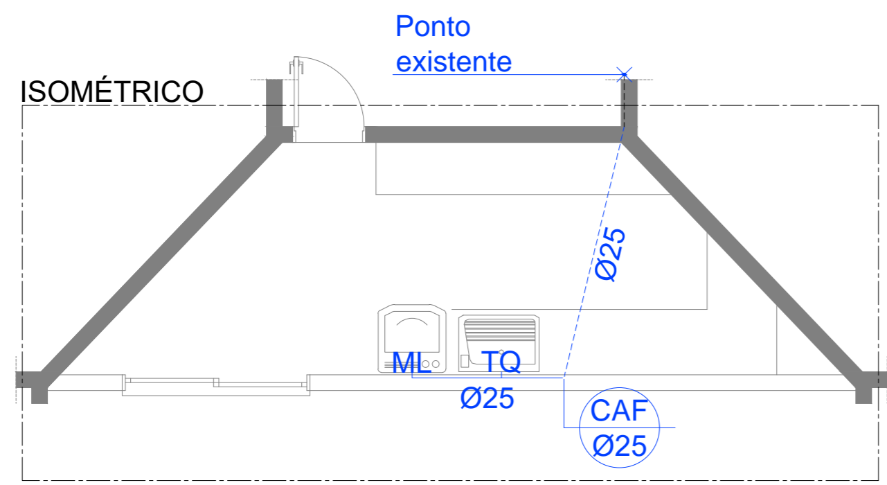
2 PROJETO DE INSTALAÇÃO DE AGUA FRIA ESC. 1:50
