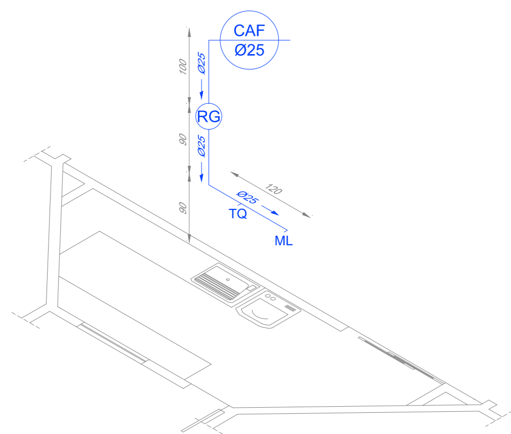
2 ESQUEMA ISOMÉTRICO ESC. 1:50
