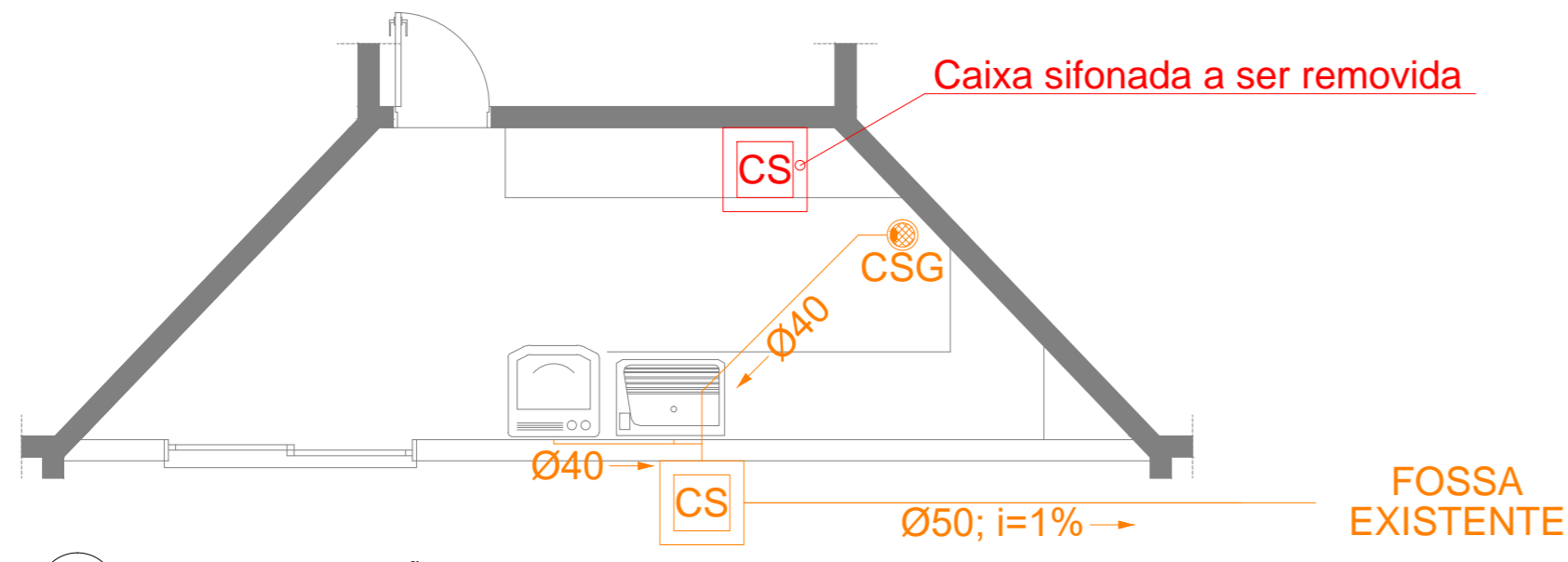
1 PROJETO DE INSTALAÇÃO DE ESGOTO ESC. 1:50
