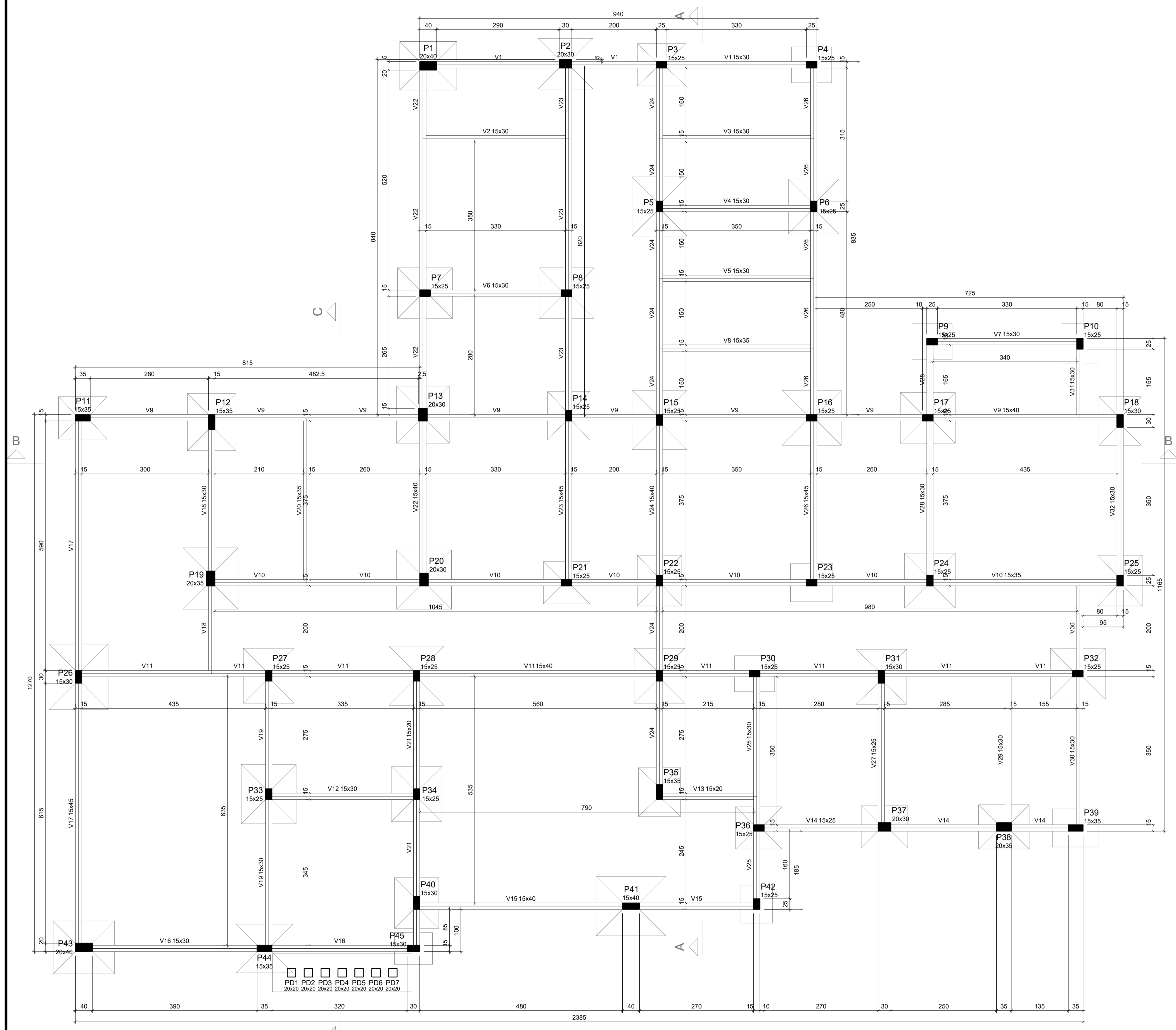
Planta de forma do pavimento térreo - nível 0 Esc: 1/50
