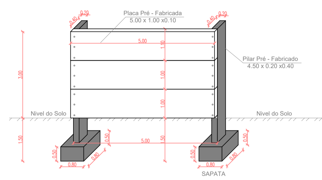
DETALHAMENTO MODULO M3 Esc: 1/75
