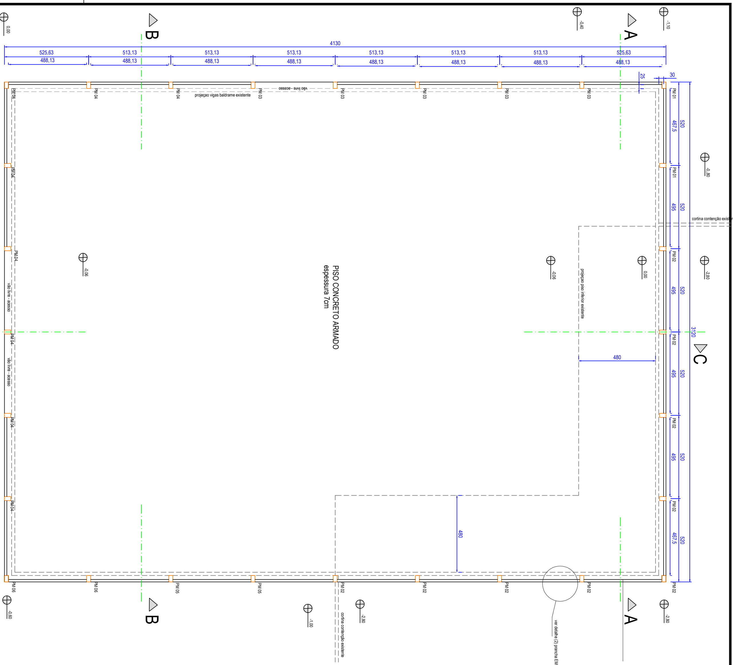
PLANTA BAIXA
